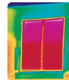
Offener Rollladen: Wärmeableitung ist hoch (rot).
